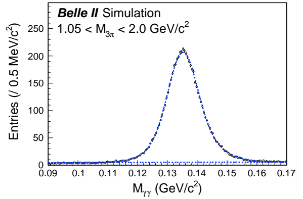
(d) 1.05 < M(3\pi) < 2.0 \text{ GeV}/c^2 (log-scale)
