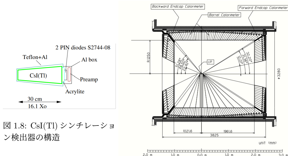
図 1.9: ECL の断面図 [10]
