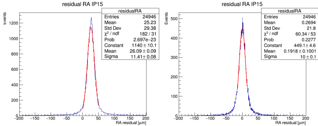
図 4.15: IP15 の並進補正前後の残差分布 (左: 補正前 x 方向、右図: 補正後 x 方向)。補正前は 26\mu\text{m} のずれがあったものが、補正後はゼロと無矛盾になっている。
