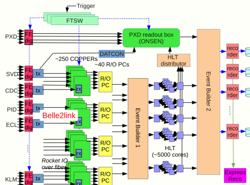
図 1.11: データ収集システムの全体図 [14]
