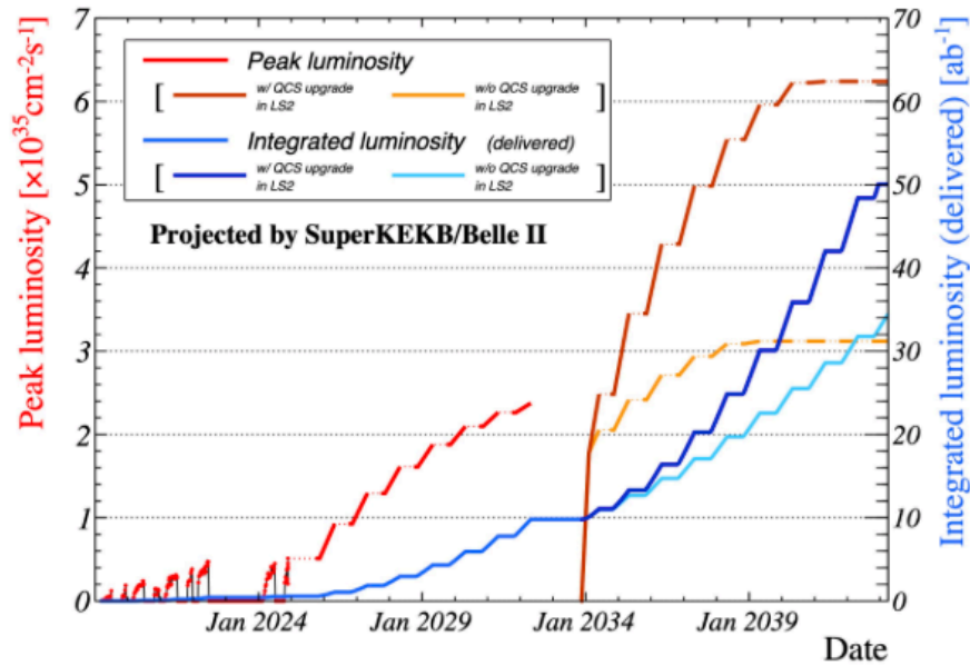
図 1.12: ルミノシティの目標値 [17]
