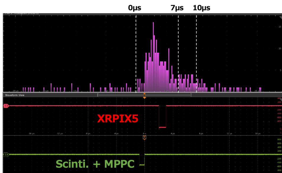
図 4.9: Trigger Latency 測定結果
