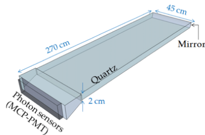
図 1.6: TOP カウンターモジュール 1 個の概形 [8]
