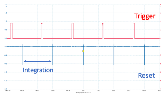
図 5.7: オシロスコープにより観測されたトリガー信号と積分タイミング。パルスレーザーが積分期間内に 1 回のみ入るよう調整されている。
