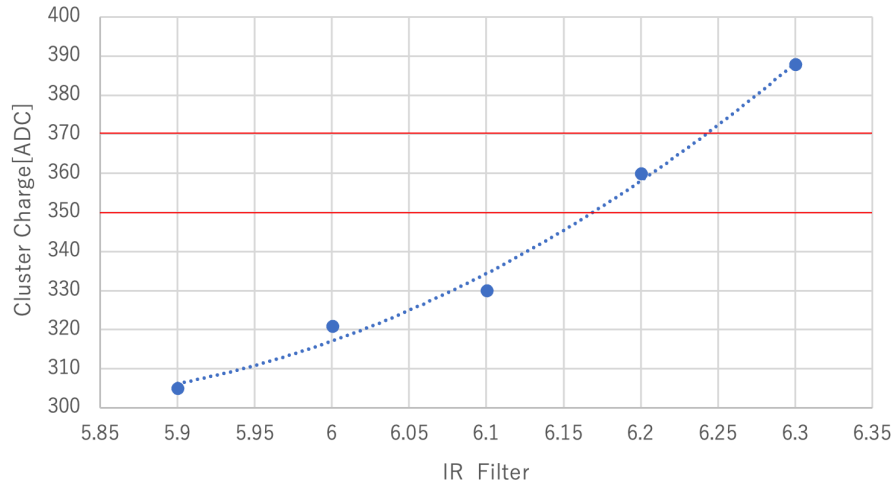
図 5.8: フィルター設定値に対するクラスタチャージの応答曲線。赤線は 1 MIP 相当の基準値 (350–370 ADC) を示す。
