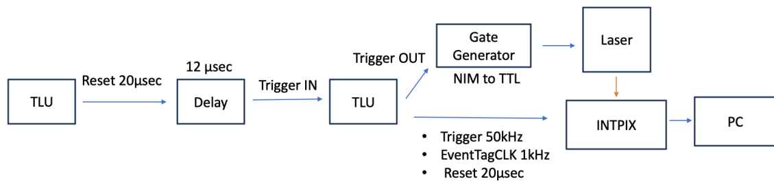
図 5.6: INTPIX4NA を用いたレーザー光量調整のセットアップ図
