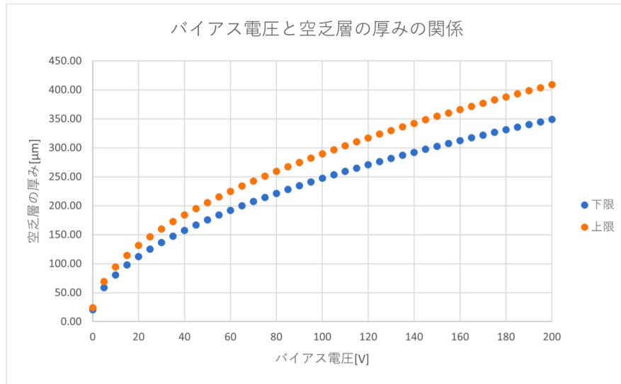
図 5.16: バイアス電圧に対する空乏層の厚みの見積り [22]
