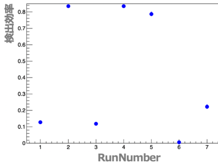
図 A.1: ALPIDE アンプ回路のパラメータを変化させた際の検出効率。Noisy および Silent Pixel は解析から除外している。パラメータ 1、3、4 では Li パラメータと同程度の検出効率が得られている一方、それ以外の設定では検出効率が著しく低下していることが確認できる。
