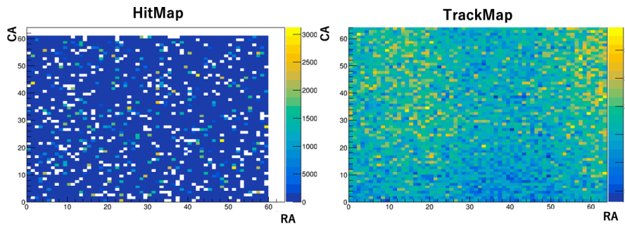
図 4.26: 合計 24 万トリガー分のヒットマップ (左) と、外挿トラックマップ (右)
