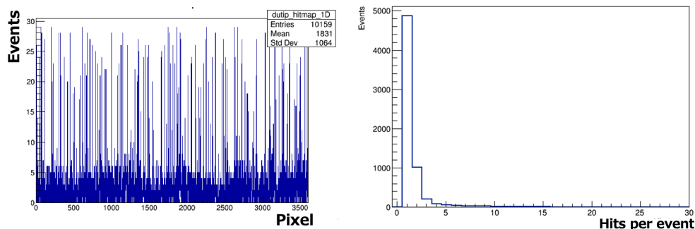
図 4.19: ノイジーピクセルをマスクした後の各ピクセルのヒット数分布 図 4.20: ノイジーピクセルをマスクした後の 1 イベントあたりのヒット数の分布
