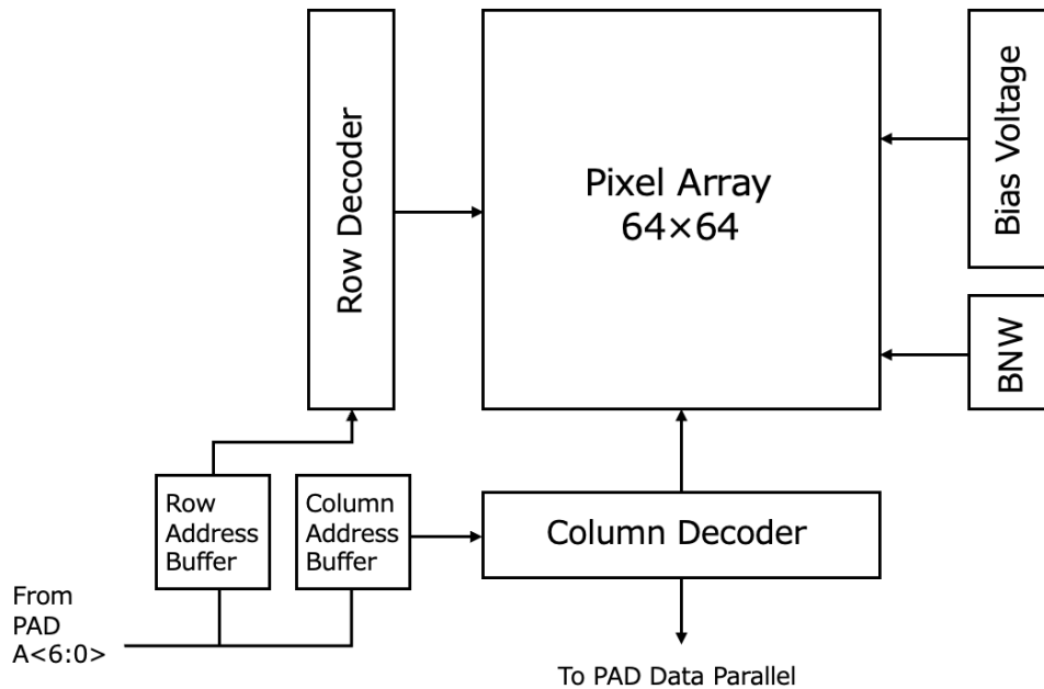
図 3.3: チップの全体構成の概略図
