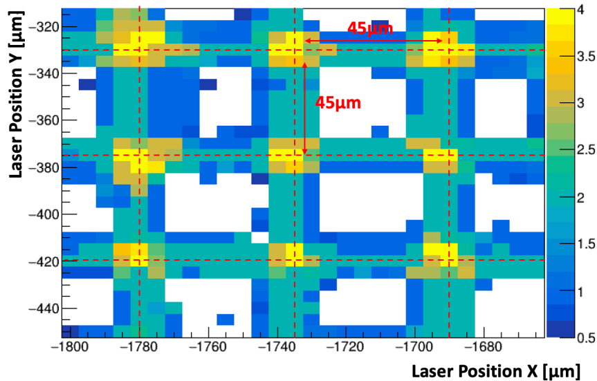
図 5.11: レーザー照射位置に対するクラスタサイズマップ
