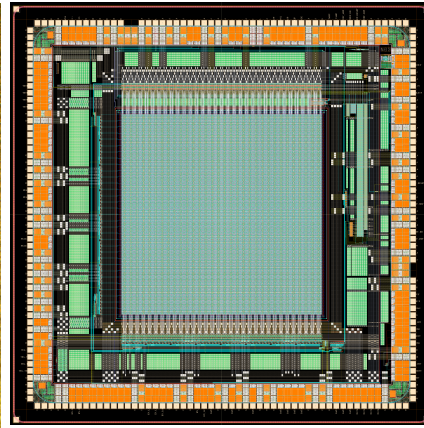
図 3.2: DuTiP1 の回路図 (CAD)
