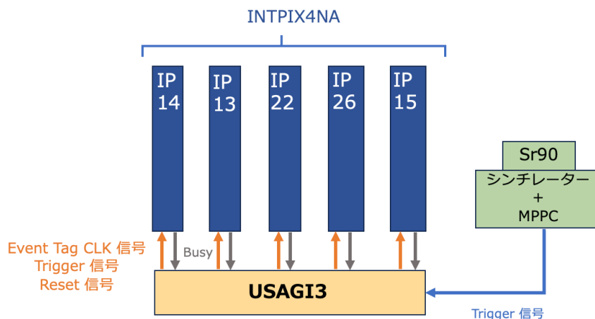
図 4.6: 同期試験のセットアップ概略図
