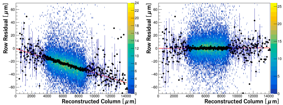
図 4.16: IP15 の回転補正前後での再構成 Column 位置と Row 方向残差の相関。赤線は一次関数によるフィッティング結果を示しており、補正後（右図）は補正前（左図）に比べて傾きが十分に小さくなっている。
