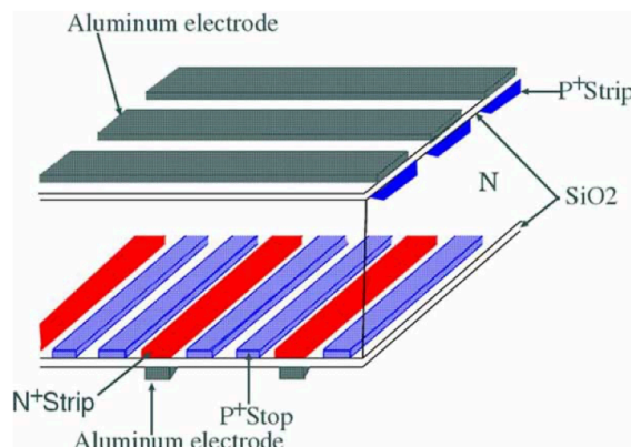
図 1.5: DSSD の構造 [6]
