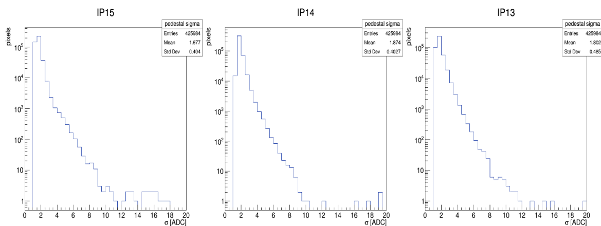
図 4.28: ペデスタル \sigma 分布
