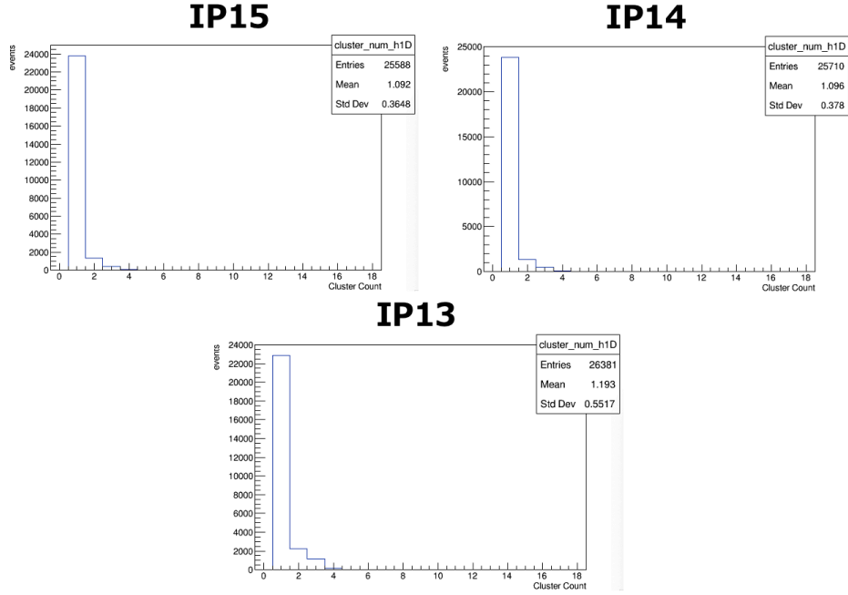
図 4.12: クラスタ数分布
