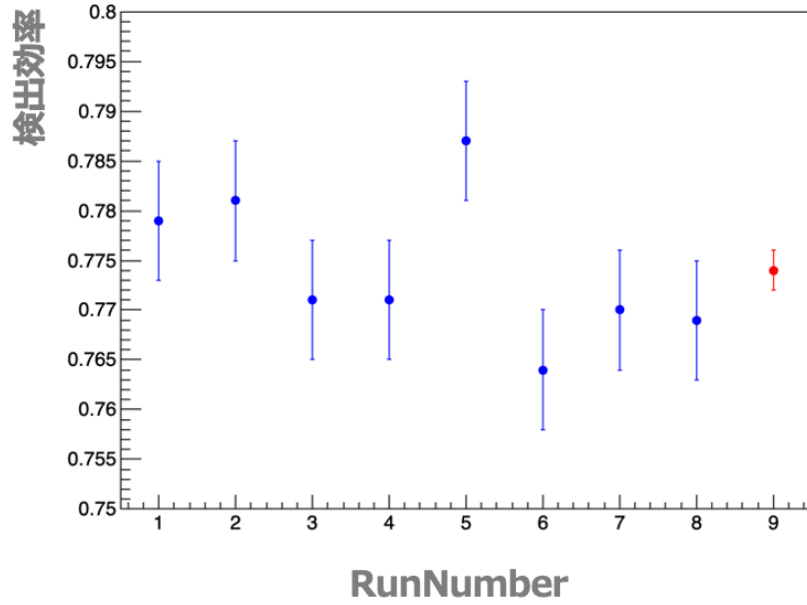
図 4.25: 各 Run における検出効率。赤点は 8 つの Run の平均値を示す。
