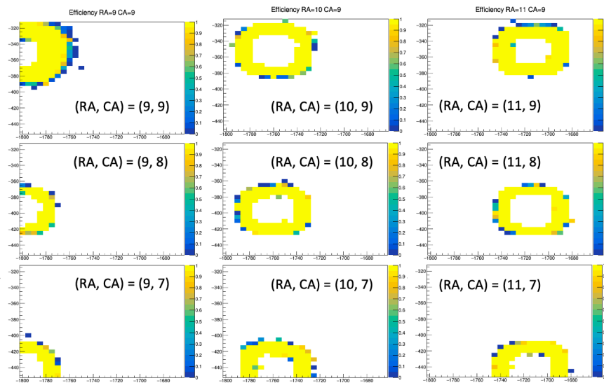
図 5.10: 3 \times 3 ピクセルにおける検出効率マップ
