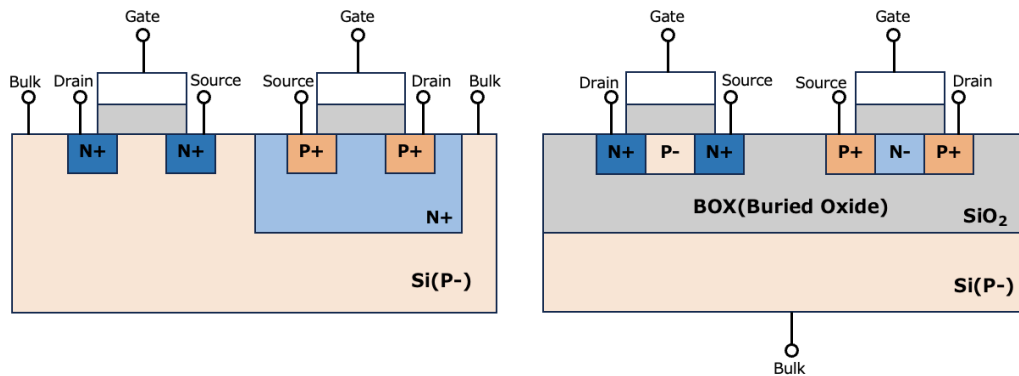
図 2.1: Bulk-CMOS(左) と SOI-CMOS(右) の構造
