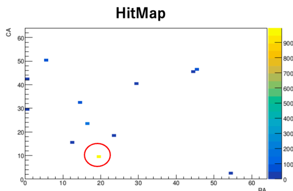
図 5.5: (RA, CA) = (20, 10) にレーザーを照射した時のヒットマップ
