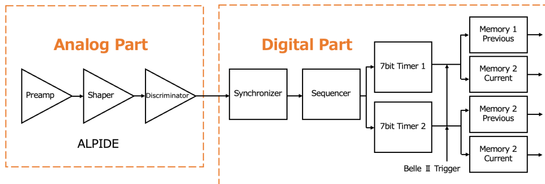
図 3.5: デジタル回路のブロック図
