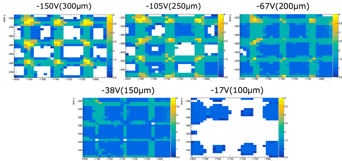
図 5.17: バイアス電圧ごとのクラスタサイズ分布
