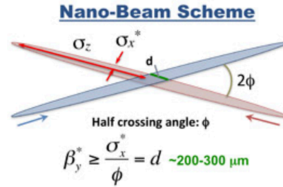
図 1.2: ナノビームスキームの概念図 [3]。陽電子バンチと電子バンチの一部が重なり、その長さが d である。このバンチの一部の交差領域で十分なルミノシティを出すよう、ビームを絞り込んだ指標となるベータ関数 \beta_y^* を d と同程度まで小さくする。
