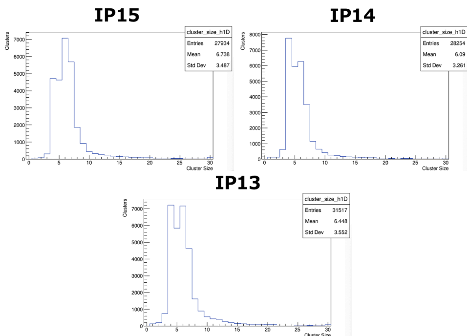
図 4.11: クラスサイズ分布
