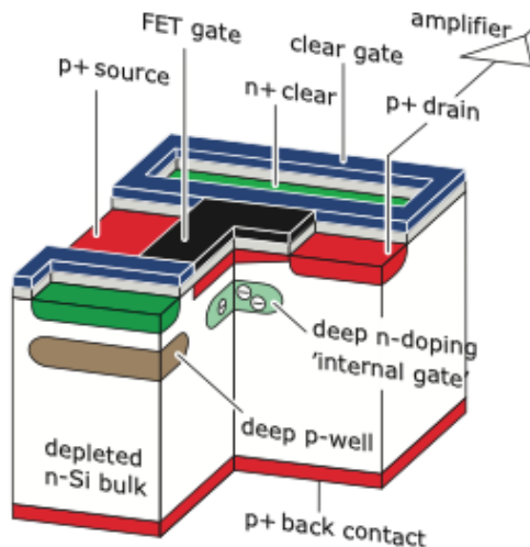
図 1.4: DEPFET の構造 [5]
