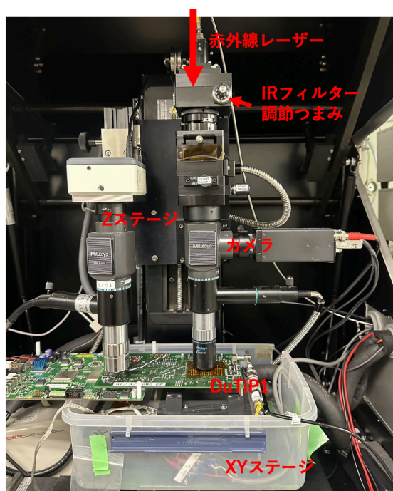
図 5.2: 実験に用いた赤外線レーザーシステムの構成
