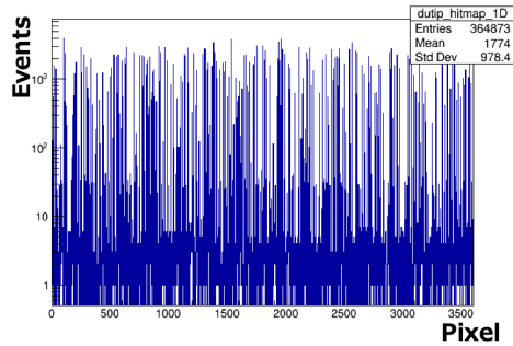
図 4.17: 各ピクセルのヒット数分布
