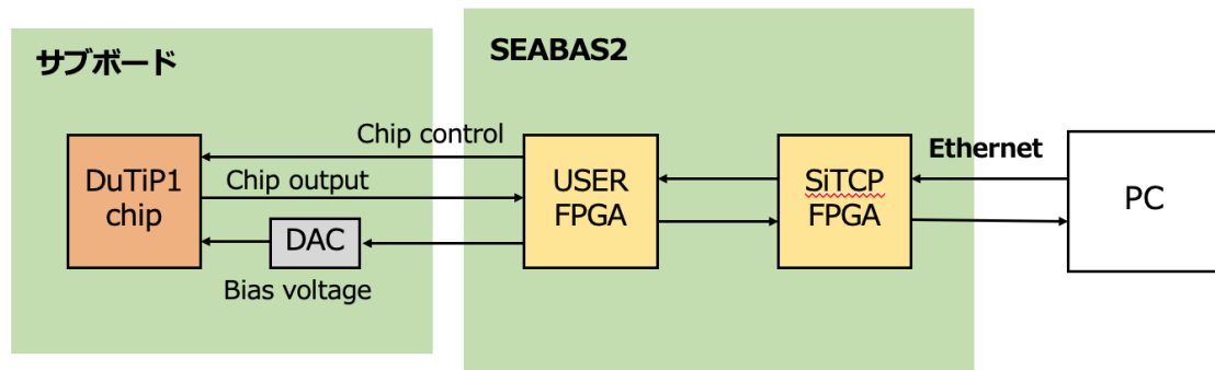
図 3.6: DuTiP1 の DAQ システムの概略図
