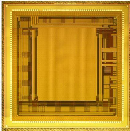
図 3.1: DuTiP1 の写真
