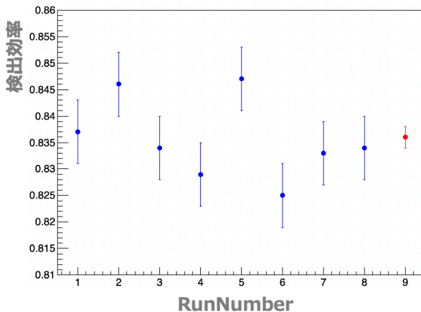
図 4.27: silent pixel を解析から除外した場合の各 Run における検出効率。赤点は 8 つの Run の平均値を示す。
