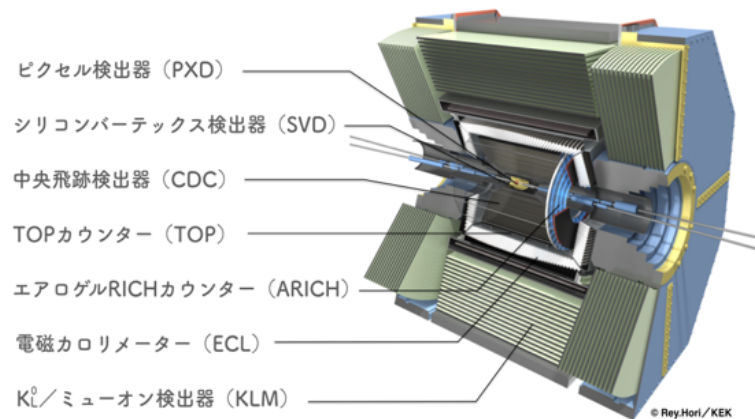
図 1.3: Belle II 測定器概要図。内部構造が分かるように一部を切り開いて描いたもの。
