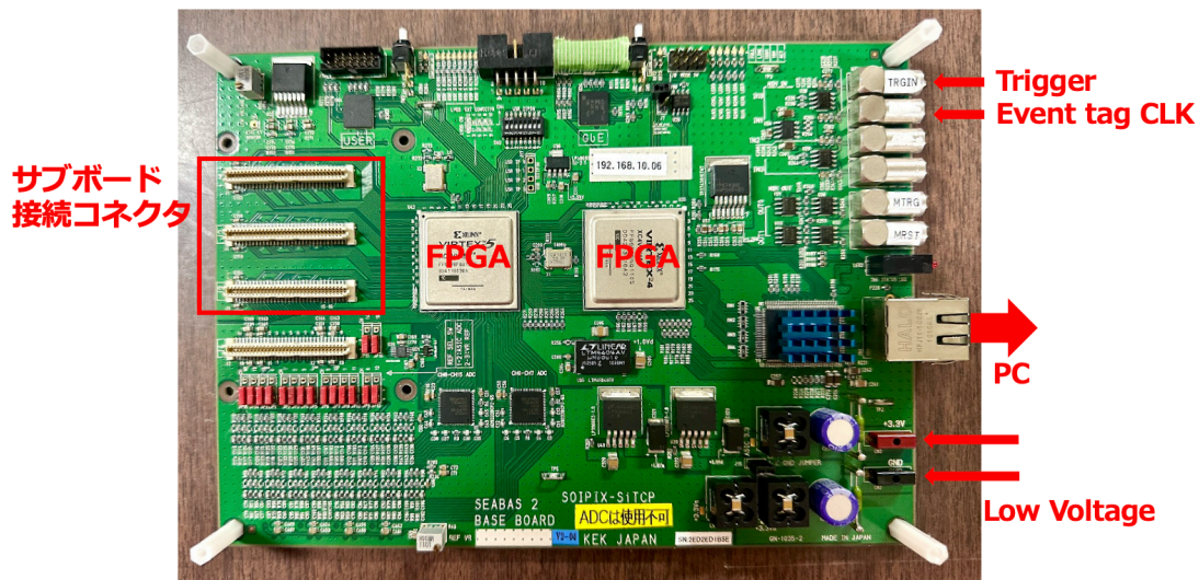
図 3.7: SEABAS 2
