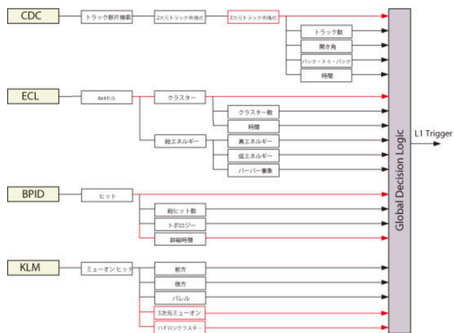
図 1.10: Belle II 実験における L1 トリガーシステムの概略図 [13]
