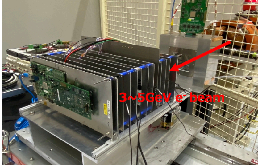
図 4.1: ビームテストのセットアップの写真。画面奥 (右上) から手前 (左下) に向けて電子ビームが到来する。エネルギーは 3 GeV から 5 GeV の範囲で可変である。
