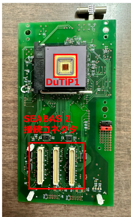
図 3.8: サブボード 表面
