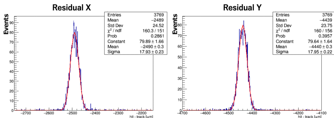
図 4.22: 並進補正前の残差分布 (左：Row 方向、 右：Column 方向)
