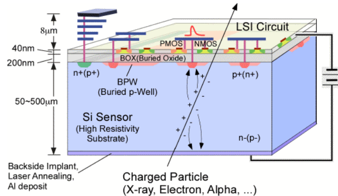
図 2.2: SOI ピクセル検出器の基本構造 [20]
