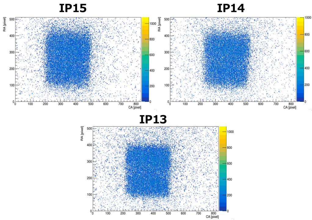
図 4.13: INTPIX4NA のヒットマップ
