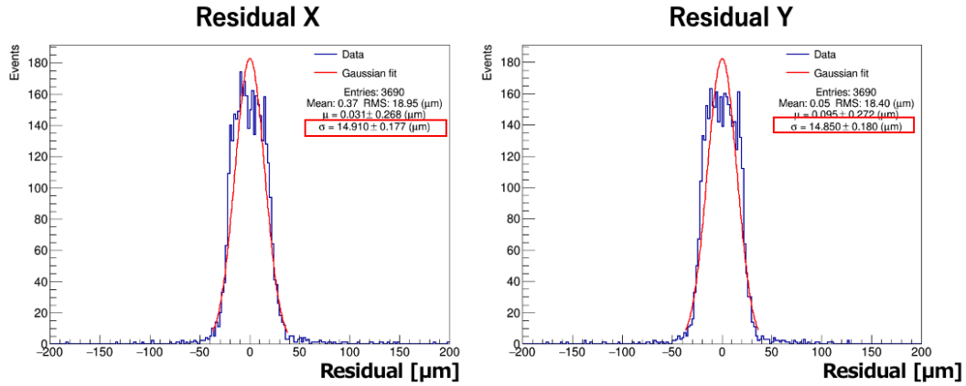
図 4.24: 残差分布（左：Row 方向，右：Column 方向）
