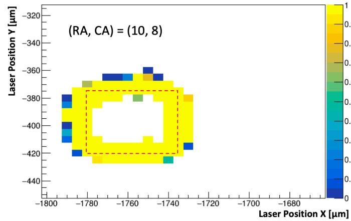
図 5.9: 単一ピクセル (RA, CA) = (10, 8) における検出効率の場所依存性。中央部に感度の低い領域が観測された。
