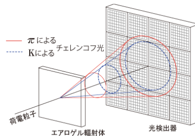
図 1.7: ARICH の識別原理 [9]
