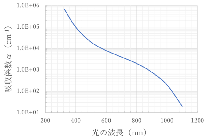
図 5.1: シリコンの光吸収係数 \alpha の波長依存性 [25]
