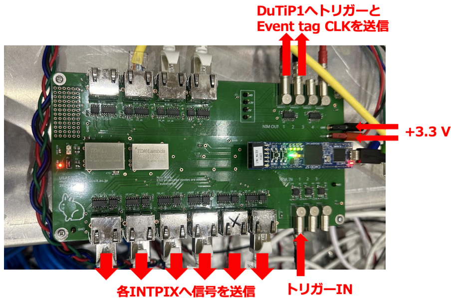
図 4.4: USAGI3 ボード
