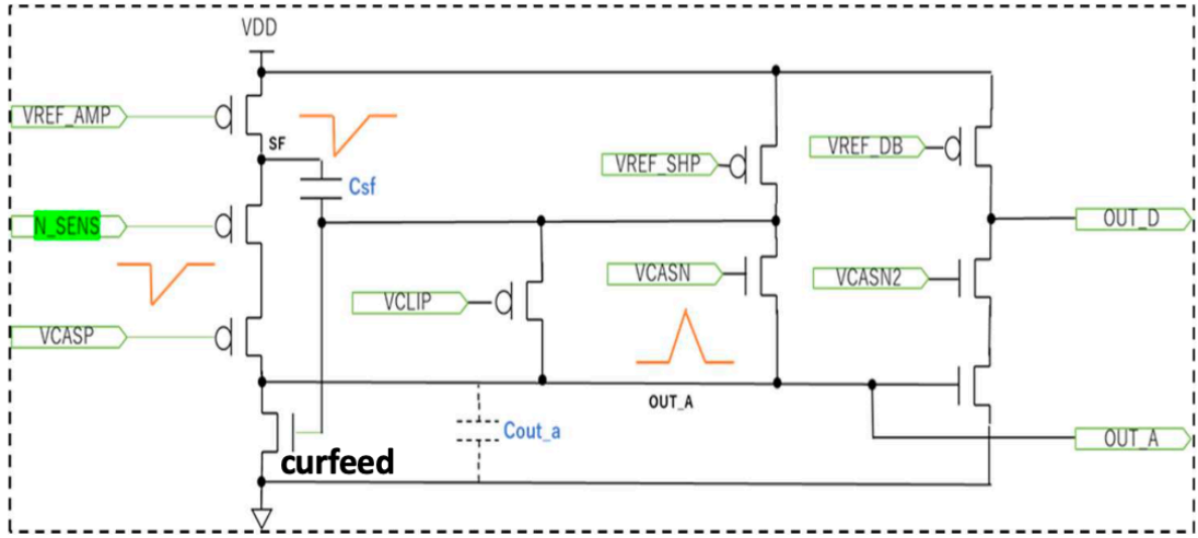
図 3.4: ALPIDE アンプの回路図
