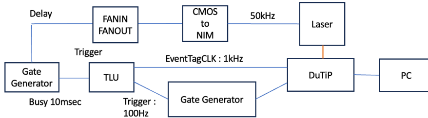
図 5.3: レーザー照射試験のセットアップ
