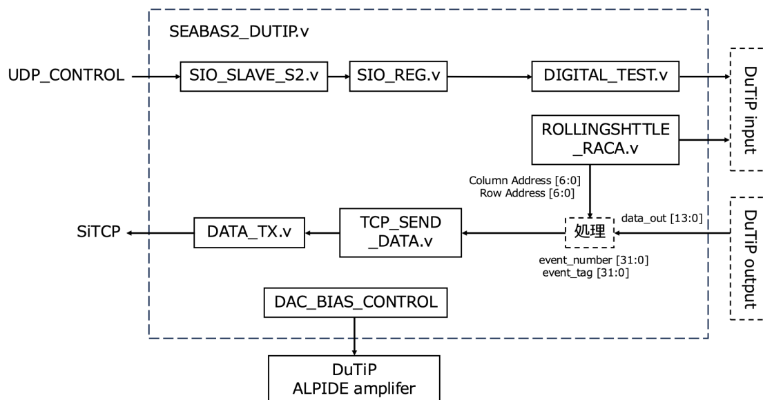
図 3.10: DuTiP1 ファームウェアのダイアグラム
