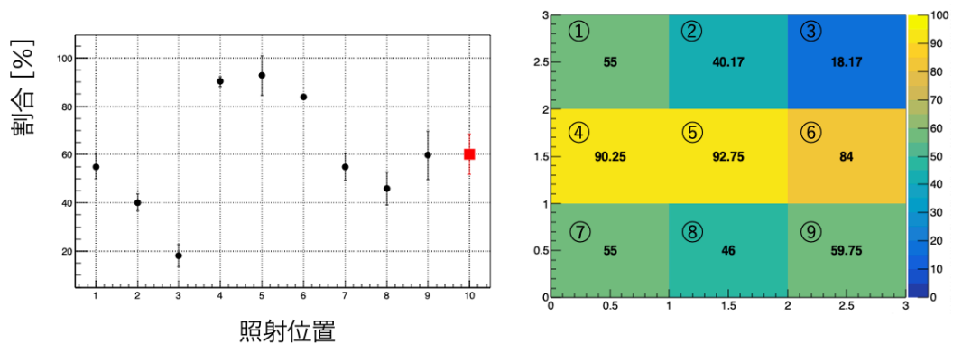
図 5.13: 各サンプルング領域における単一ピクセル応答に基づく不感領域の割合。数値はピクセル面積に対する非検出領域のパーセンテージを示す。左図の赤点は 9 領域の平均値を示したものである。
