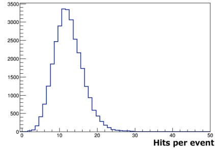
図 4.18: 1 イベントあたりのヒット数分布
