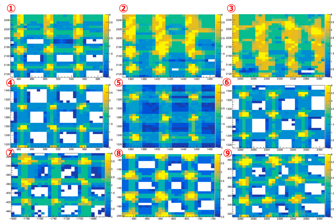
図 5.14: 各サンプリング領域におけるクラスタサイズ分布
