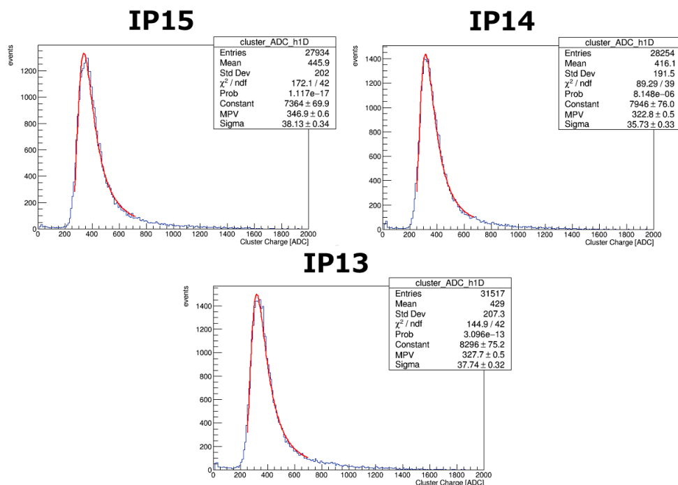
図 4.10: クラスチャージ分布。単位は ADC カウント
