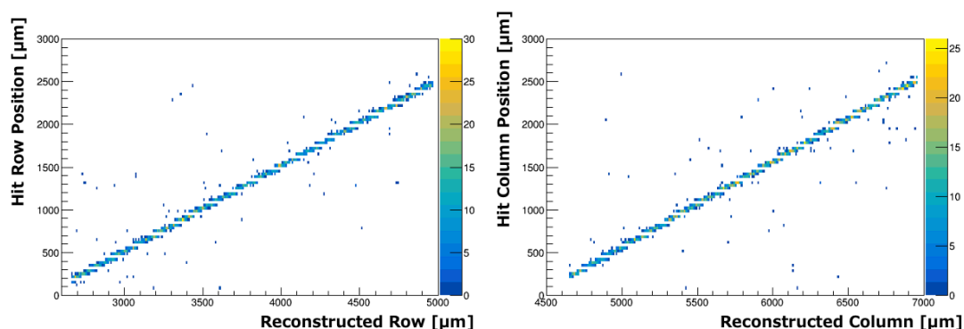
図 4.21: ヒット位置とトラック位置の相関 (左: Row 方向、右: Column 方向)
