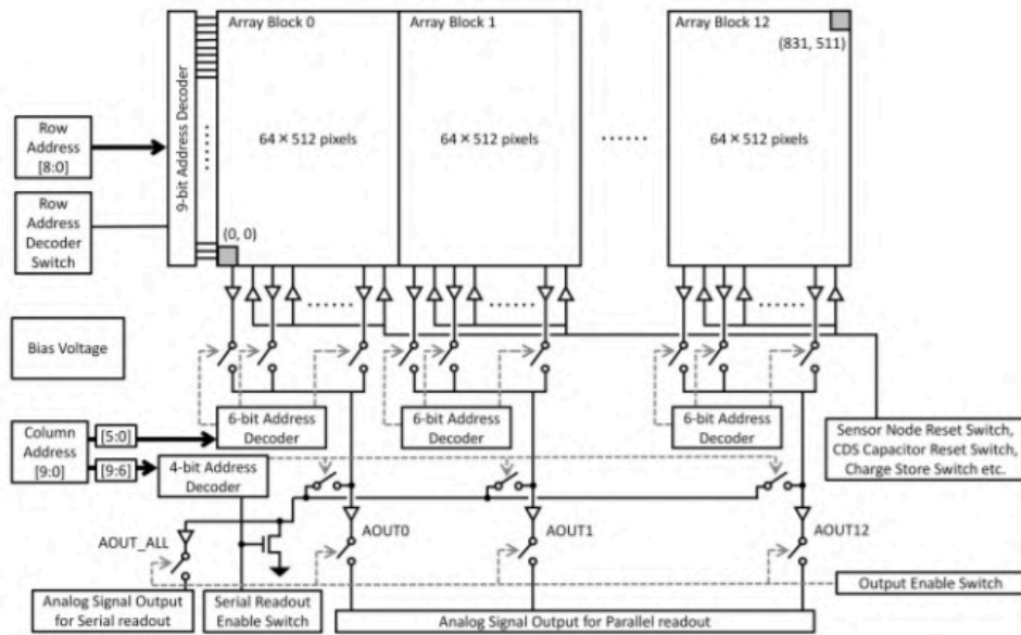
図 4.3: INTPIX4NA の IO-Path[24]
