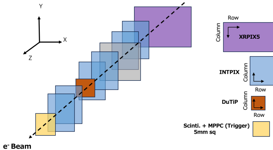
図 4.2: ビームテストのセットアップの概略図
