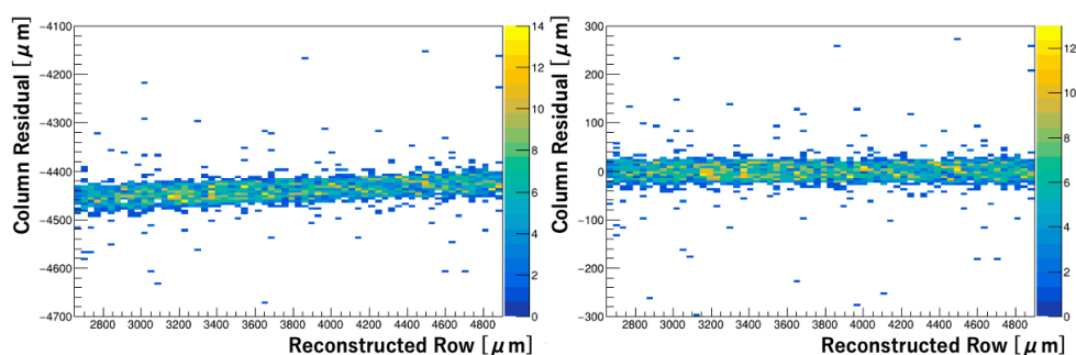
図 4.23: 回転補正前後での再構成した Row 方向位置と Column 方向残差の相関
