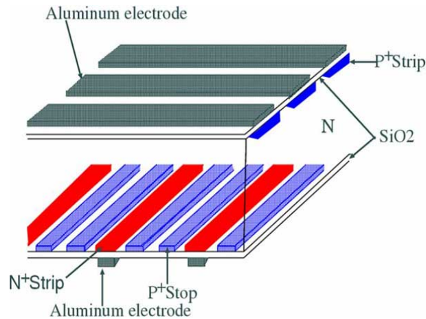
図 2.8: DSSD の構造 [10]
