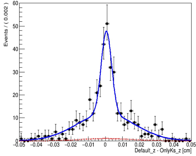
図 6.5: 実験データの \Delta z' 分布。本文中に記したフィット結果の線を描きこんでいる。
