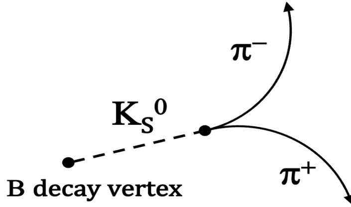
図 3.1: B 中間子から K_S^0 \rightarrow \pi^+ \pi^- への過程
