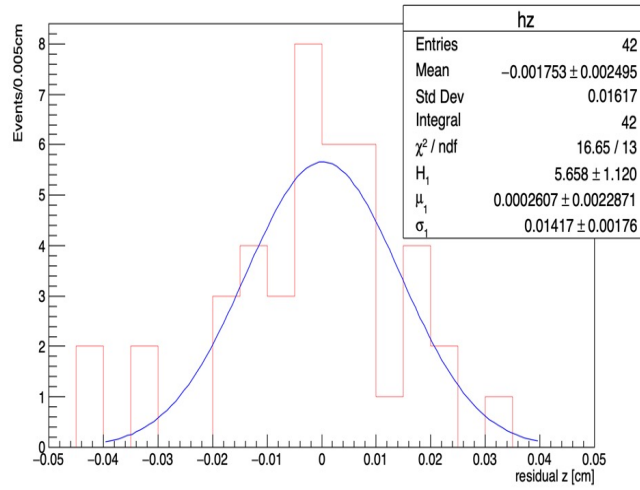
図 6.4: 実験データの背景事象の \Delta z' 分布。本文中に記したフィット結果の線を描きこんでいる。
