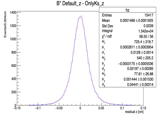
図 1.15: \Delta z' 分布 (first hit が Layer5)
