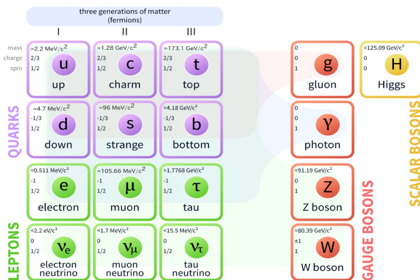
図 1.1: 標準理論での素粒子の種類 [1]
