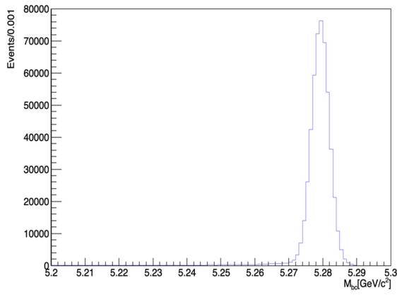
図 4.6: signalMC の M_{\text{bc}} 分布
