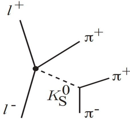
図 4.1: B^+ \rightarrow J/\psi K^{*+}(\rightarrow K_S^0 \pi^+) 崩壊
