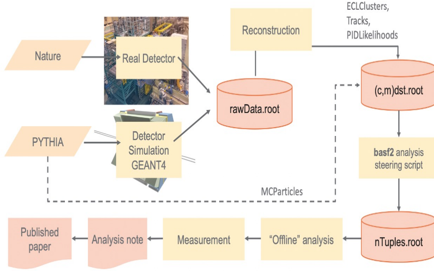
図 4.2: データ取得からデータ解析、論文になるまでの流れ [30]
