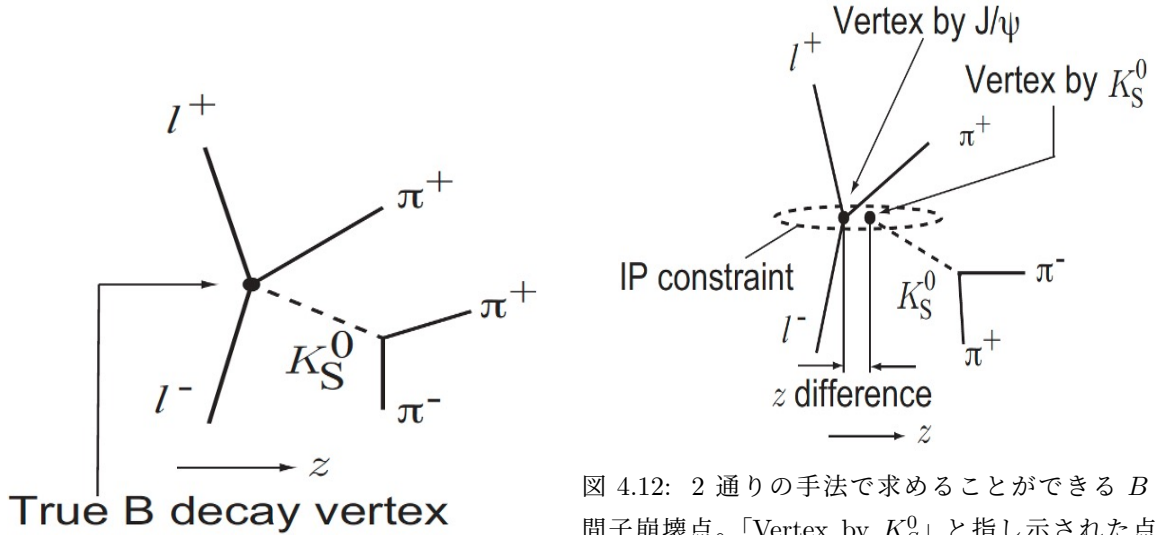
図 4.11: B^+ \rightarrow J/\psi K^{*+} (\rightarrow K_S^0 \pi^+) 崩壊では B 中間子 K_S^0 \rightarrow \pi^+ \pi^- から IP に向けて逆向きに外挿して求め子の真の崩壊点と同一地点で J/\psi も K^{*+} も崩壊する。 図 4.12: 2 通りの手法で求めることができる B 中間子崩壊点。「Vertex by K_S^0 」と指し示された点が B 中間子の崩壊点で、「Vertex by J/\psi 」と指し示された点が J/\psi \rightarrow \mu^+ \mu^- から求める B 中間子の崩壊点である。
