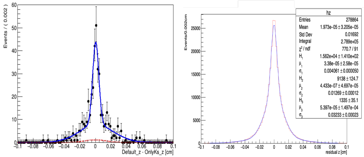
図 2.1: 実験データの \Delta z' 分布 (フィット範囲 : \pm 0.1\text{cm} ) 図 2.2: シミュレーションサンプルの \Delta z' 分布 (フィット範囲 : \pm 0.1\text{cm} )
