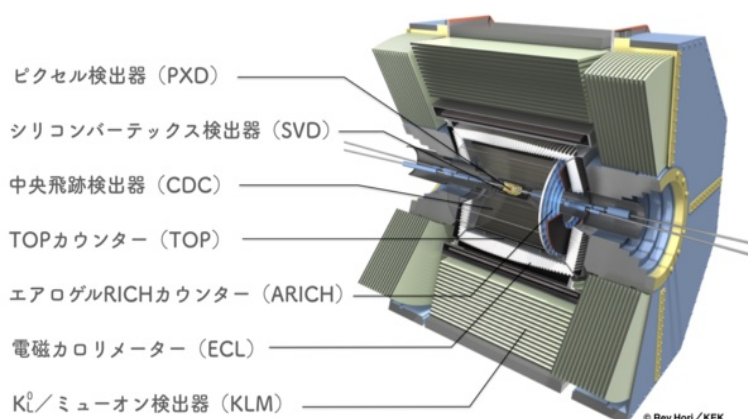
図 2.3: Belle II 測定器の概要図
