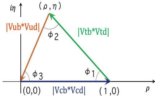
図 1.2: ユニタリティ三角形
