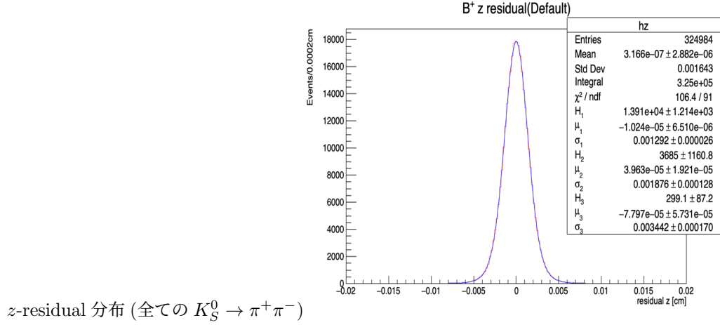
図 1.11: \Delta z' 分布 (全ての K_S^0 \rightarrow \pi^+\pi^- )
