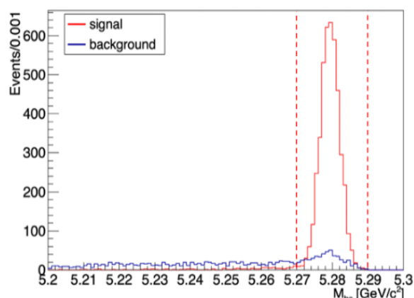
図 5.1: signalMC における -0.06 \text{ GeV} < \Delta E < 0.04 図 5.2: signalMC における 5.27 \text{ GeV}/c^2 < M_{bc} < 5.29 \text{ GeV} の M_{bc} 分布。期待される信号事象の分布も 5.28 \text{ GeV}/c^2 の範囲の \Delta E 分布。期待される信号事象の \text{GeV}/c^2 のピークとして描きこまれている。分布も 0 \text{ GeV} のピークとして描きこまれている。
