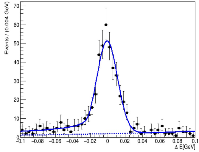
図 6.3: 実験データの \Delta E 分布 ( 5.27\text{GeV}/c^2 < M_{bc} < 5.29\text{GeV}/c^2 かつ -0.1\text{ GeV} < \Delta E < 0.1\text{ GeV} )。フィット結果の線が描きこまれている。
