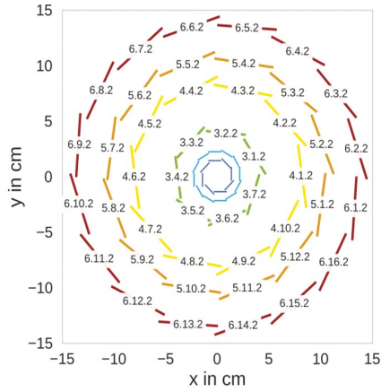
図 2.4: VXD のシリコンピクセルセンサーおよびシリ コンストリップセンサー配置の xy 平面投影図。 図 2.5: VXD の Layer の配置。 rz 平面内で描いたもの。縦横比は同一スケールではない。
