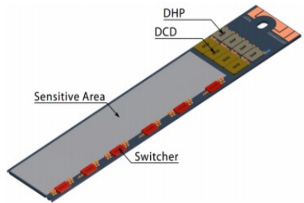
図 2.7: DEPFET
