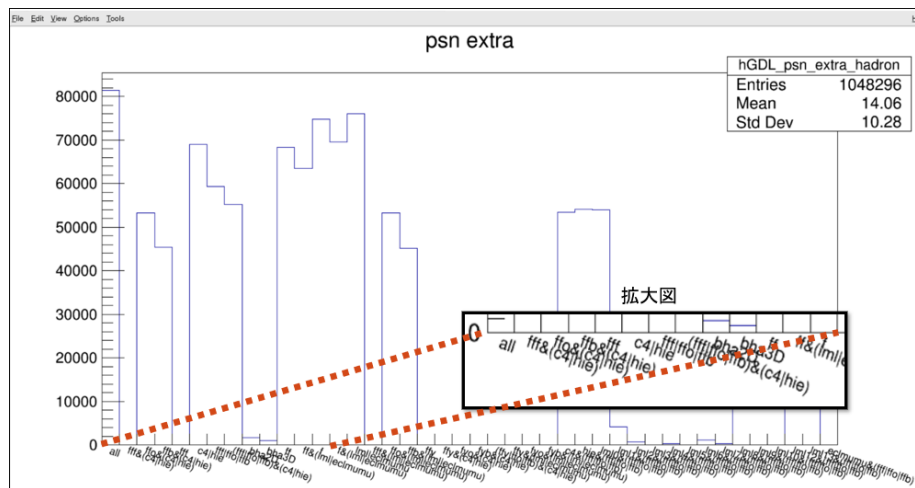
図 94 DAQHLLTヒストグラムの図
