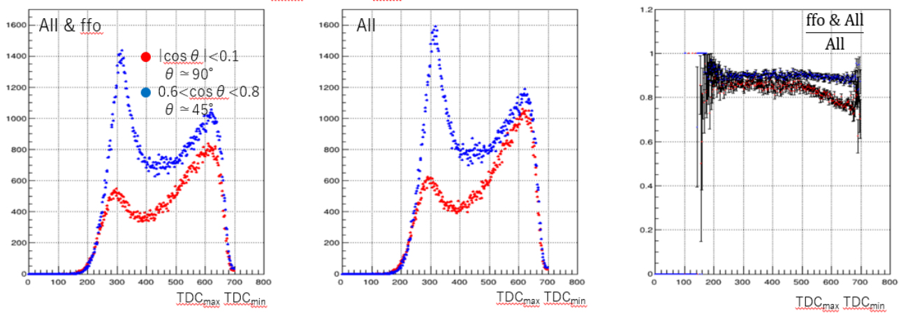
図 115 T_{max} - T_{min} の分布
